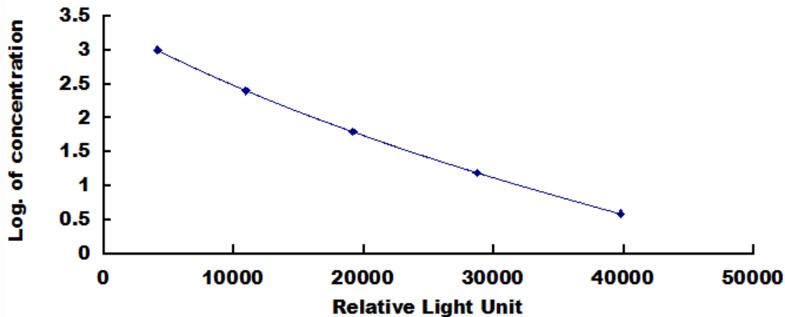
多巴胺 (DA) 检测试剂盒标准曲线
