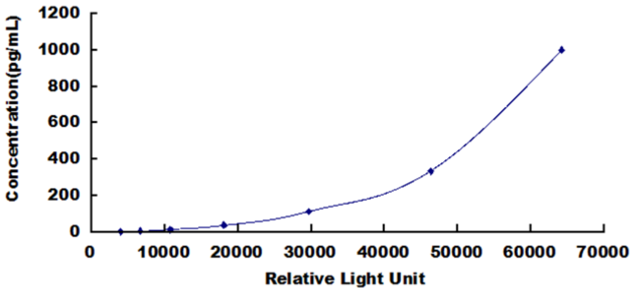
人白介素 17 (IL17) 检测试剂盒标准曲线
