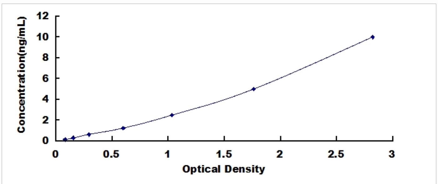
钠/钾离子转运 ATP 酶 \alpha 1 肽 (ATP1 \alpha 1 ) 检测试剂盒标准曲线
