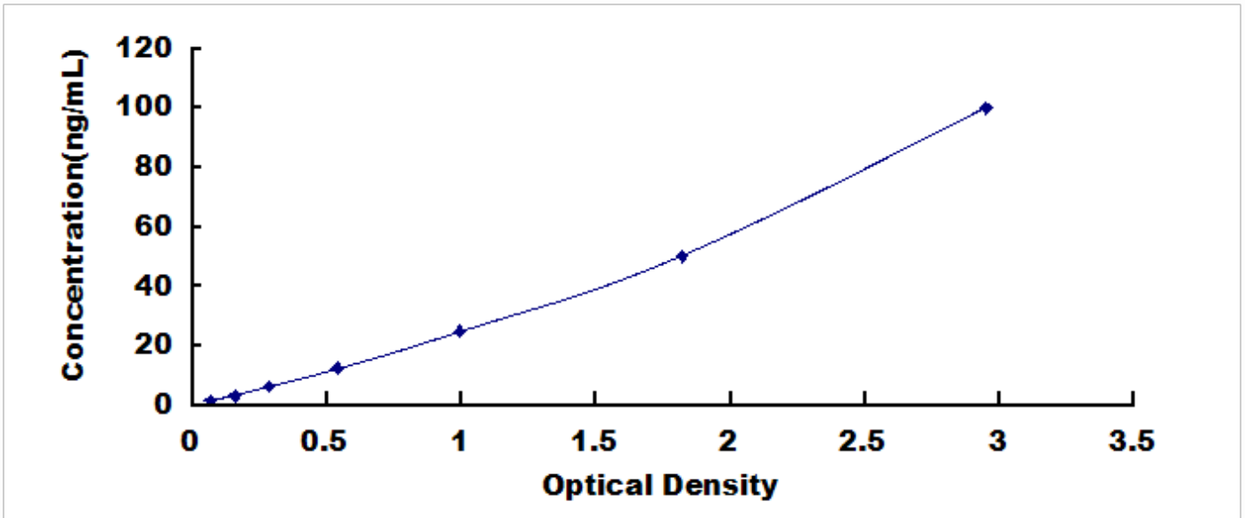
人脂肪酸酰胺水解酶 (FAAH) 检测试剂盒标准曲线
