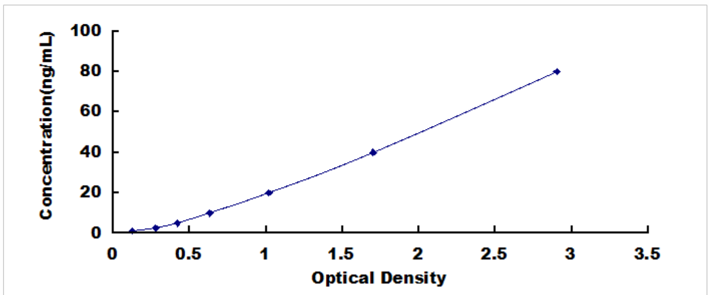
人 \alpha 1-抗胰糜蛋白酶 ( \alpha 1ACT) 检测试剂盒标准曲线
