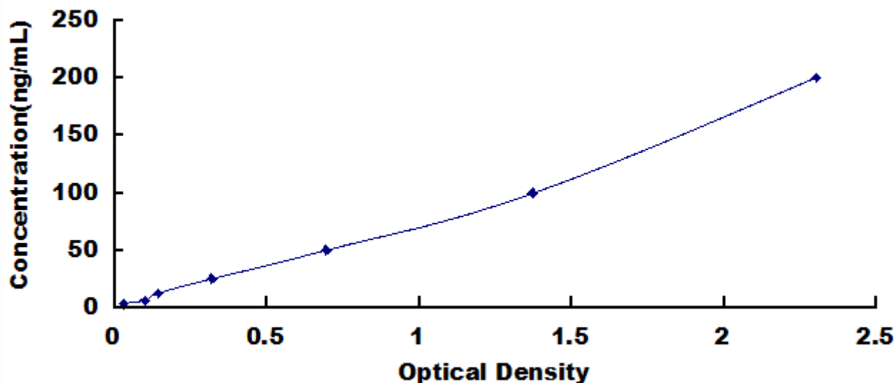
抗绿色荧光蛋白抗体(Anti-GFP)检测试剂盒标准曲线
