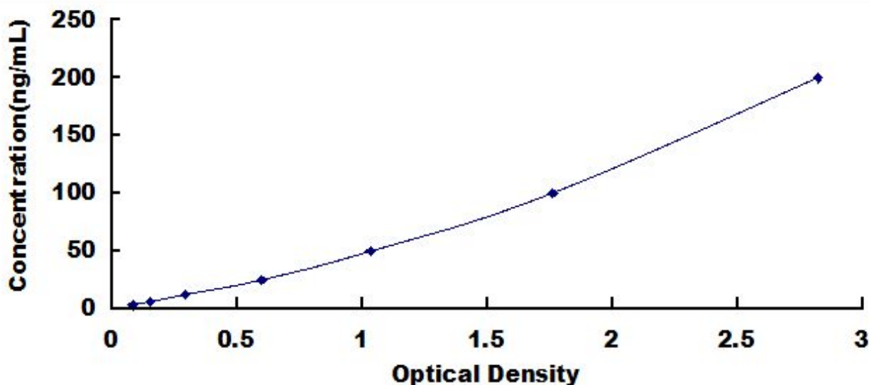
人抗髓鞘碱性蛋白抗体(Anti-MBP)检测试剂盒标准曲线
