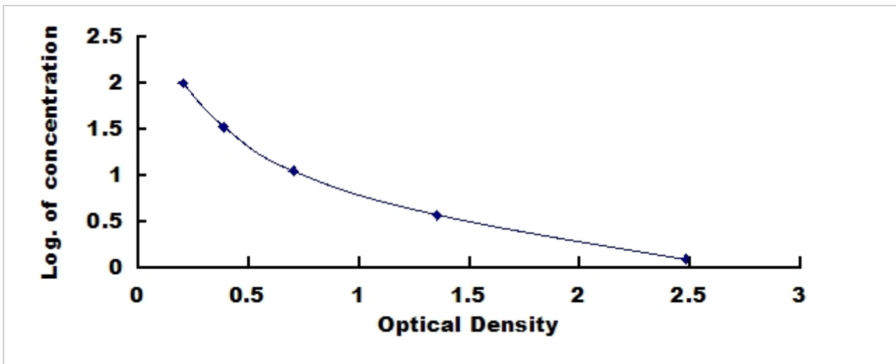
牛抑肽酶(AP)检测试剂盒标准曲线
