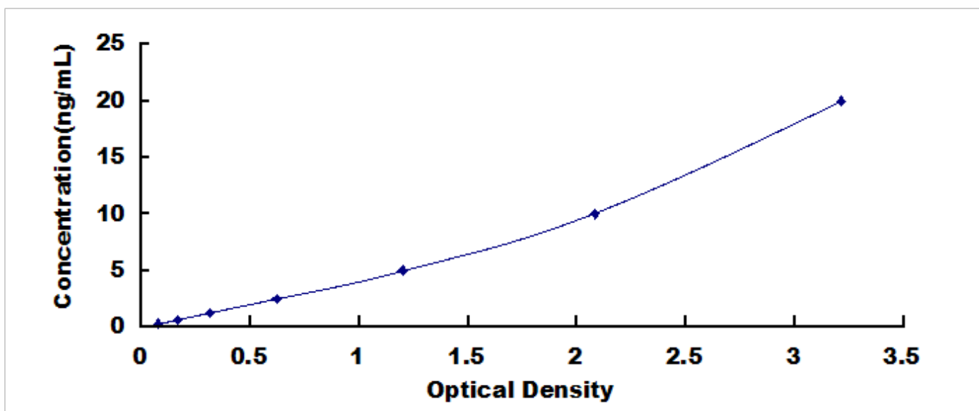
人胆绿素还原酶 B (BLVRB) 检测试剂盒标准曲线
