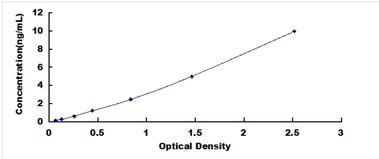
犬 C 反应蛋白 (CRP) 检测试剂盒标准曲线
