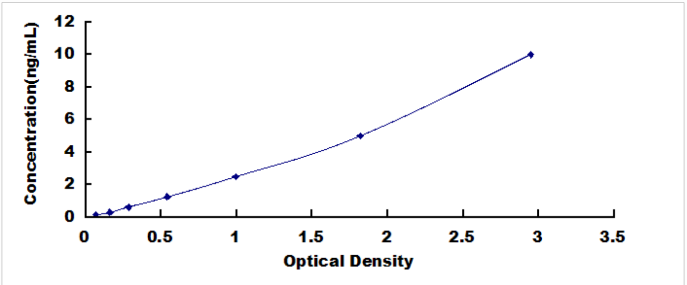
人 CD8a 分子 (CD8a) 检测试剂盒标准曲线
