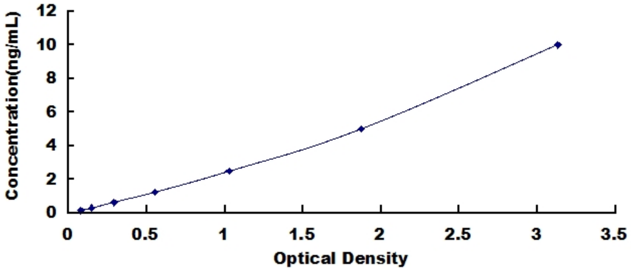
人 Crk 样蛋白 (CRKL) 检测试剂盒标准曲线
