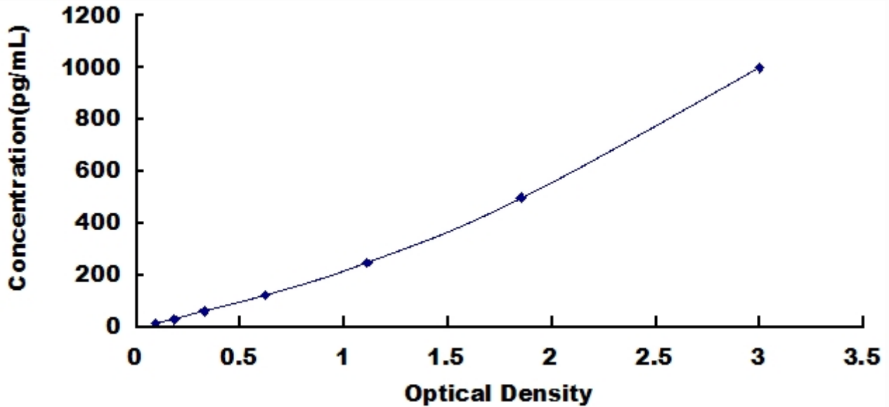
犬半胱氨酸蛋白酶抑制剂 3 (CST3) 检测试剂盒标准曲线
