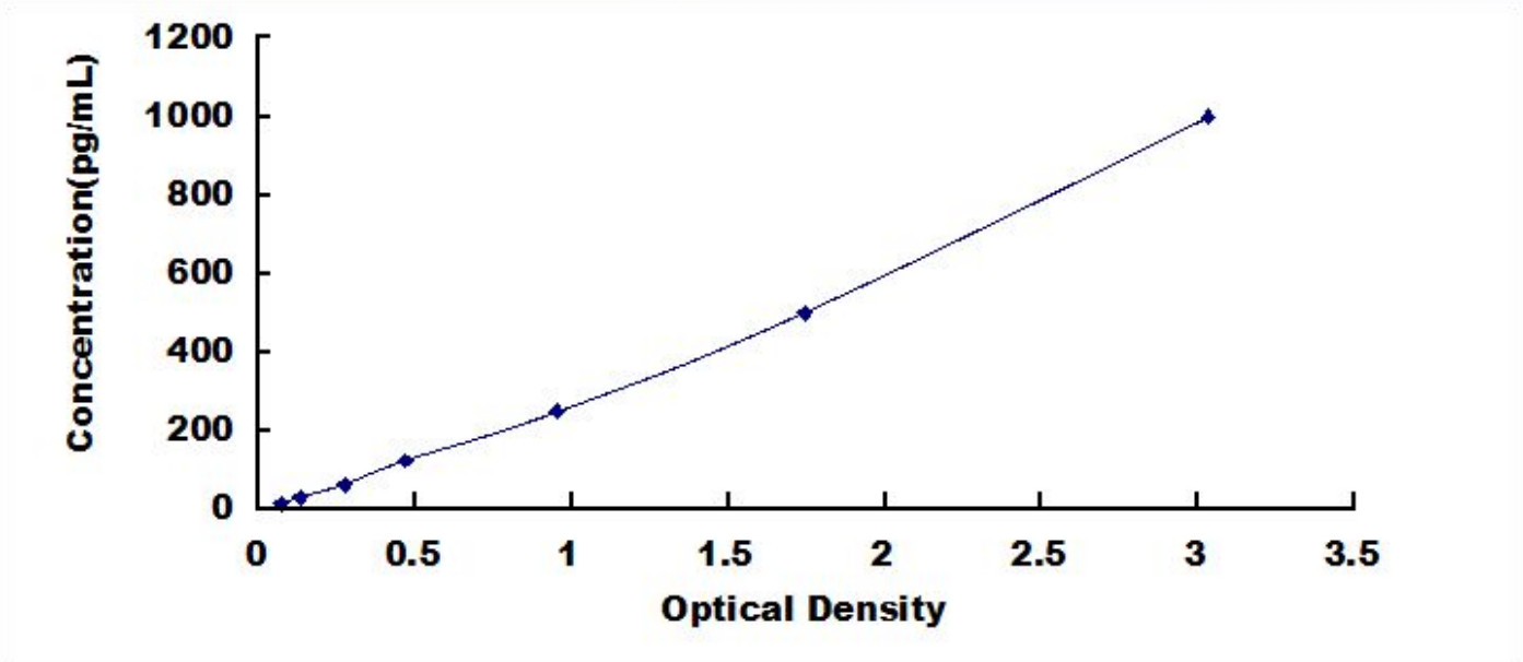
大鼠表皮生长因子(EGF)检测试剂盒标准曲线
