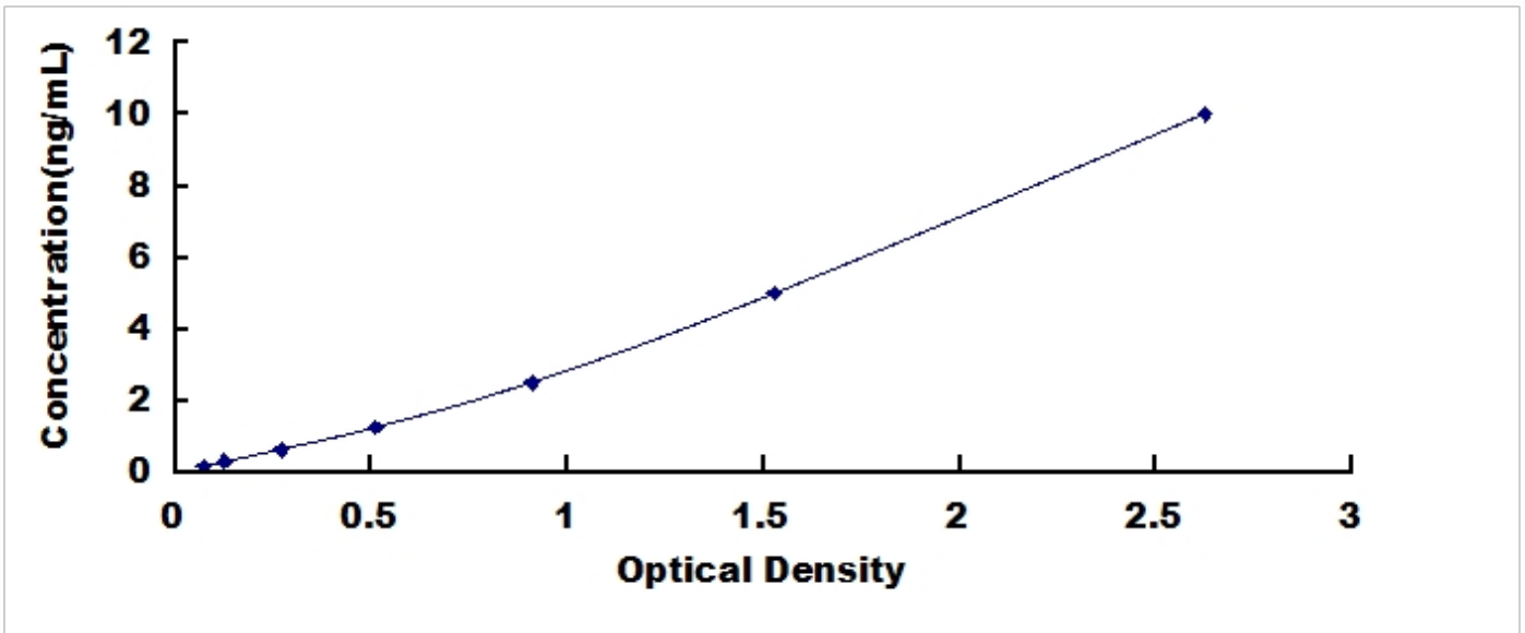
大鼠葡萄糖转运蛋白 4 (GLUT4) 检测试剂盒标准曲线
