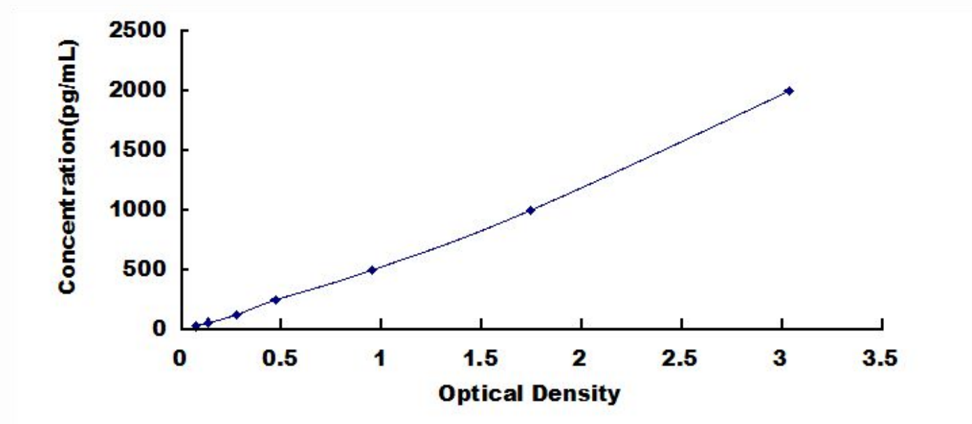
小鼠血红素氧合酶 1 (H01) 检测试剂盒标准曲线
