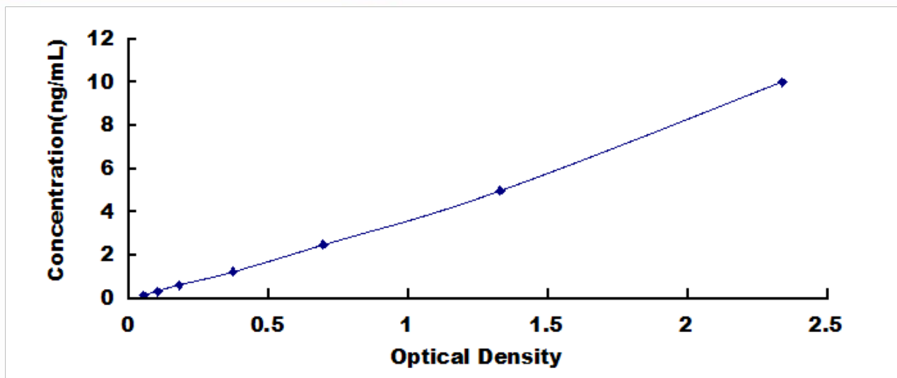
大鼠胰岛素样生长因子 1 (IGF1) 检测试剂盒标准曲线
