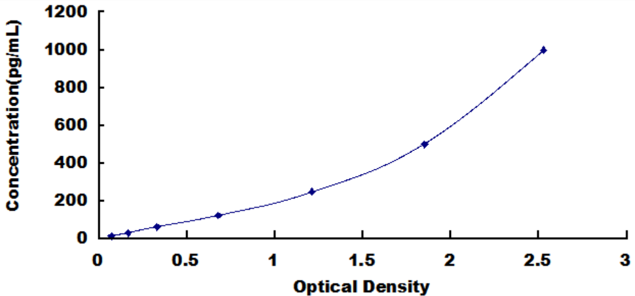
小鼠干扰素 β (IFN β) 检测试剂盒标准曲线
