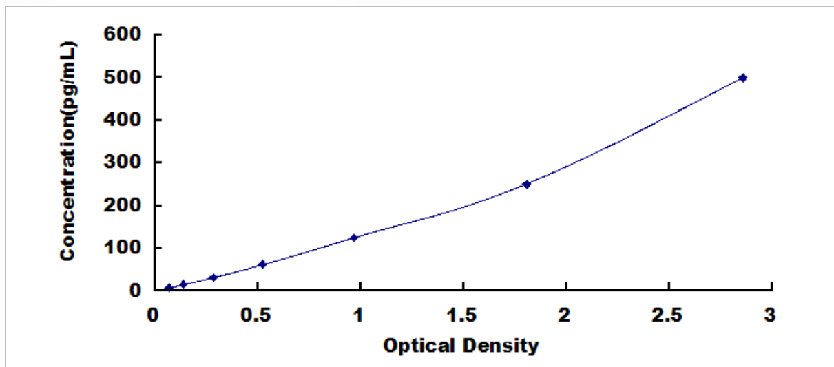
小鼠白介素 23 (IL23) 检测试剂盒标准曲线
