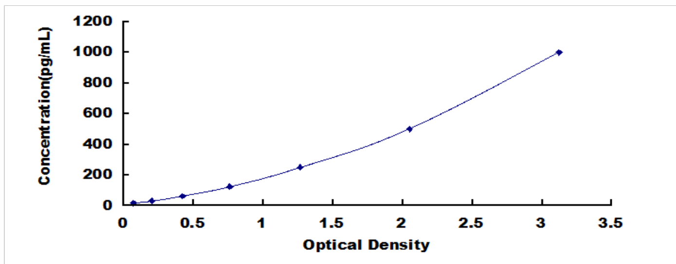
小鼠白介素 28A (IL28A) 检测试剂盒标准曲线
