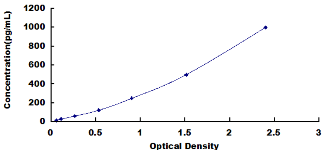
猪白介素 5 (IL5) 检测试剂盒标准曲线
