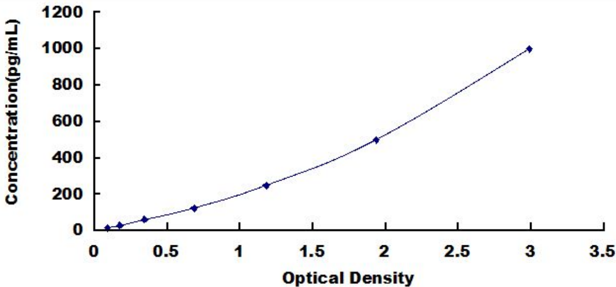
小鼠巨噬细胞炎性蛋白 3 \alpha (MIP3 \alpha ) 检测试剂盒标准曲线
