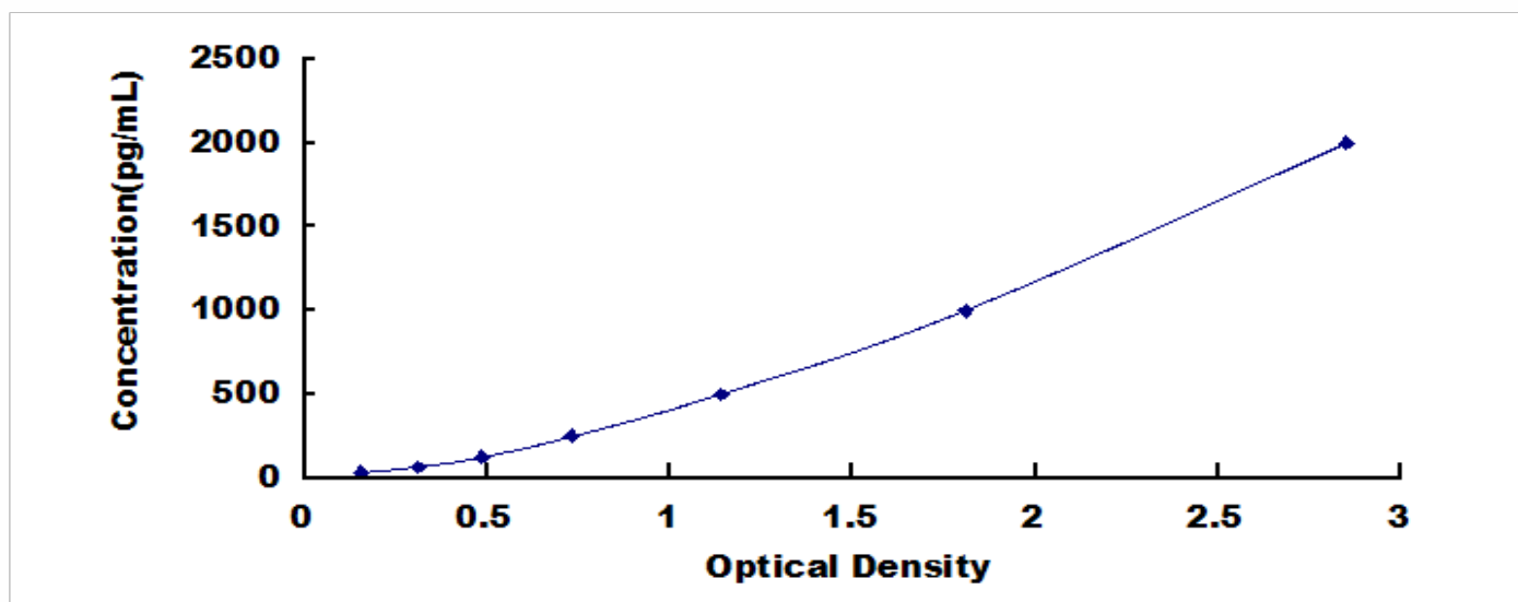
人干扰素 \gamma 诱导单核因子 (MI \gamma ) 检测试剂盒标准曲线
