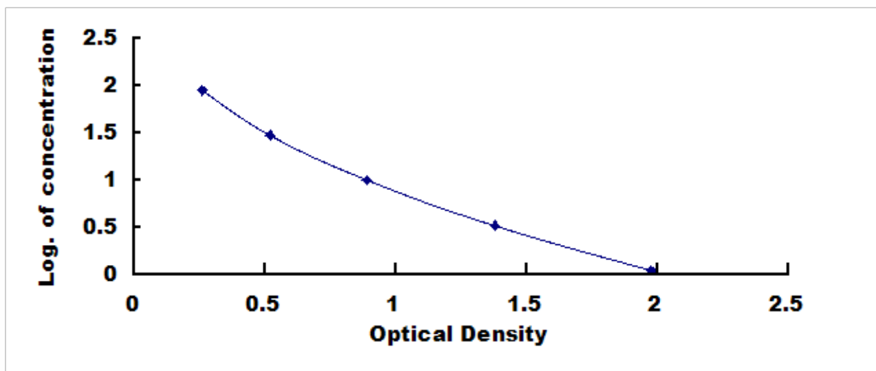
大鼠肌肉生长抑制素 (MSTN) 检测试剂盒标准曲线
