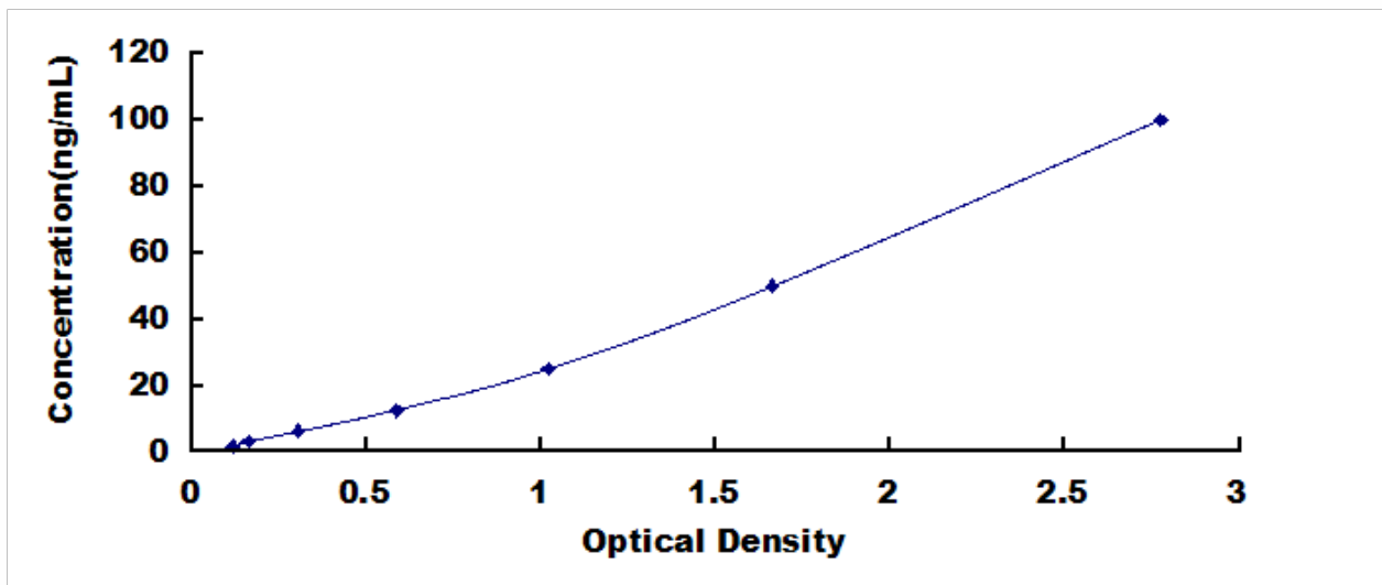
人神经细胞黏附分子 (NCAM) 检测试剂盒标准曲线
