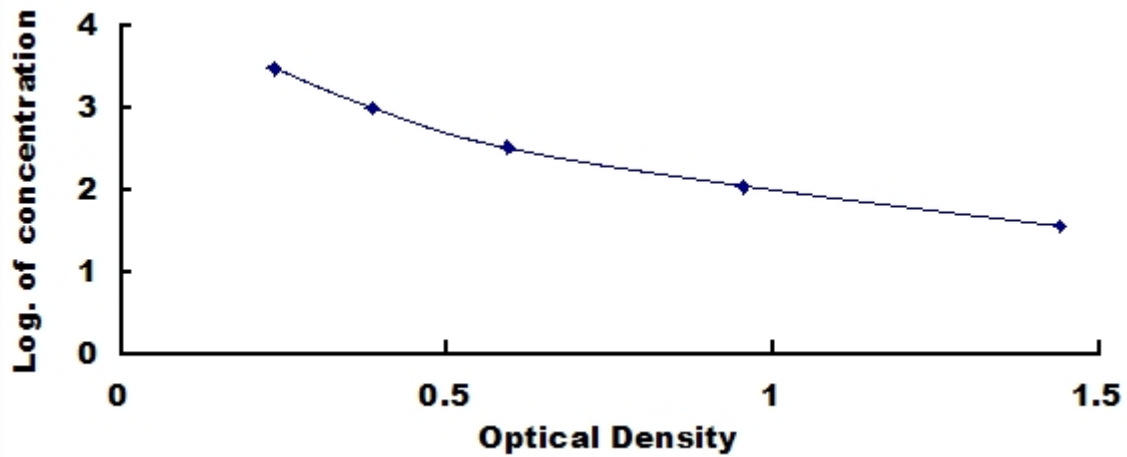
小鼠神经降压素 (NT) 检测试剂盒标准曲线
