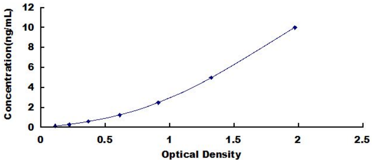
人核有丝分裂器蛋白 1 (NUMA1) 检测试剂盒标准曲线
