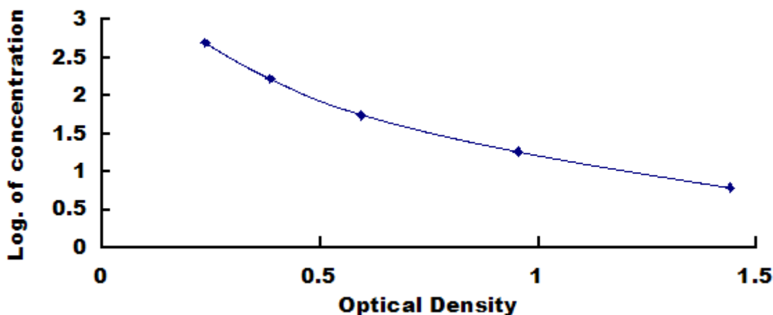
磷脂酰肌醇三磷酸 (PIP3) 检测试剂盒标准曲线
