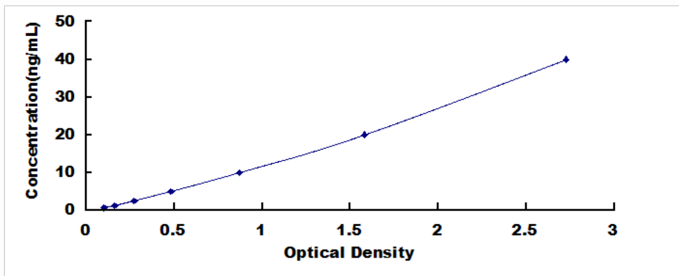
人脂蛋白关联磷脂酶 A2 (LpPLA2) 检测试剂盒标准曲线
