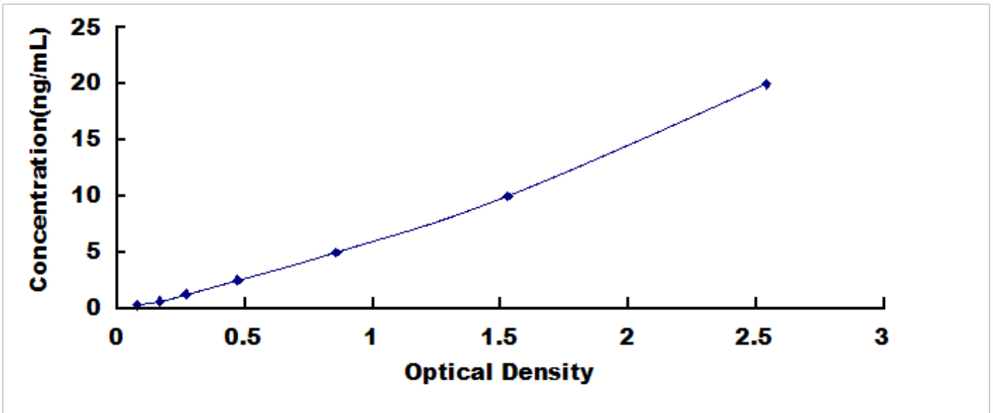
大鼠甲状腺过氧化物酶(TPO)检测试剂盒标准曲线
