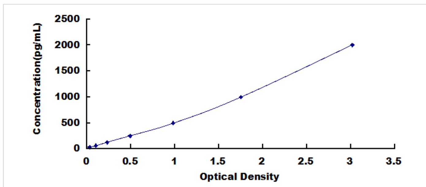
人三叶因子 2(TFF2)检测试剂盒标准曲线
