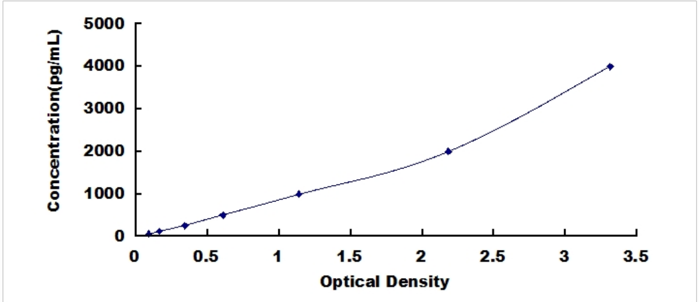
人三叶因子 3 (TFF3) 检测试剂盒标准曲线
