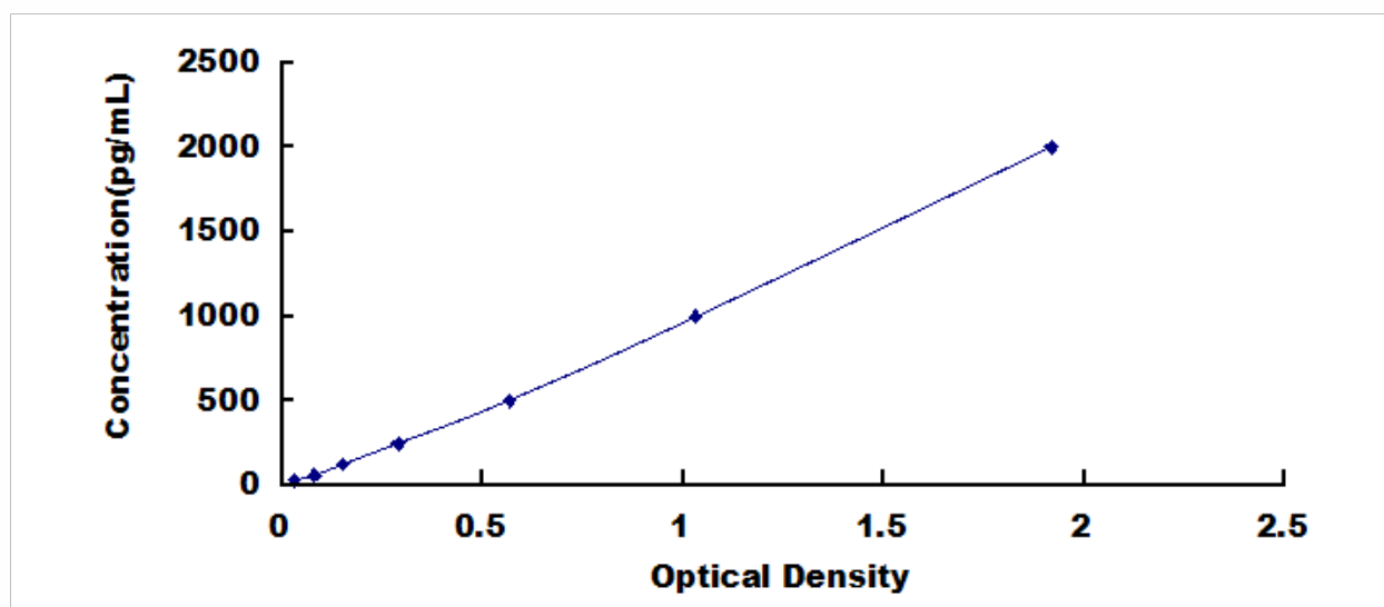
人类胰蛋白酶(TPS)检测试剂盒标准曲线
