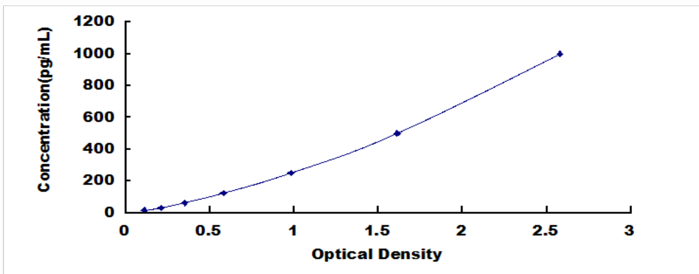
山羊肿瘤坏死因子 \alpha (TNF \alpha ) 检测试剂盒标准曲线
