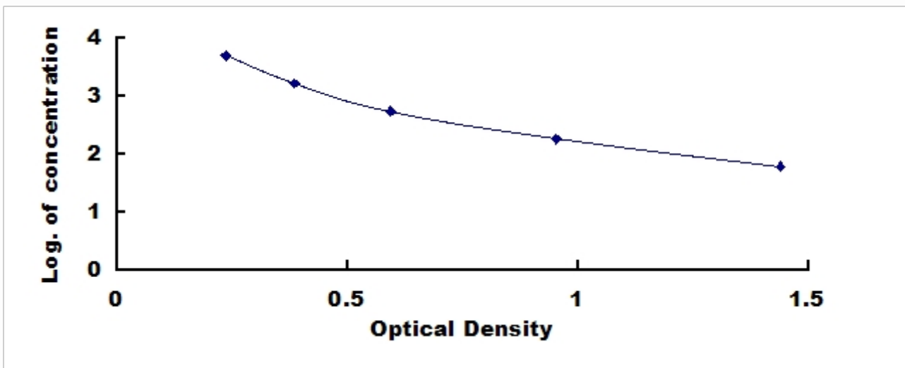
尿苷三磷酸 (UTP) 检测试剂盒标准曲线
