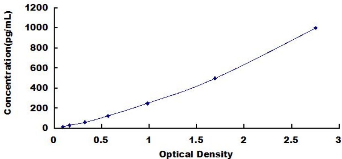
兔血管内皮生长因子 A (VEGFA) 检测试剂盒标准曲线
