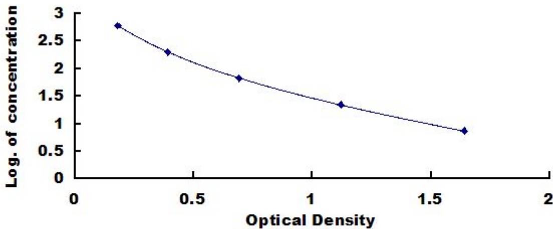
维生素 B2 (VB2) 检测试剂盒标准曲线
