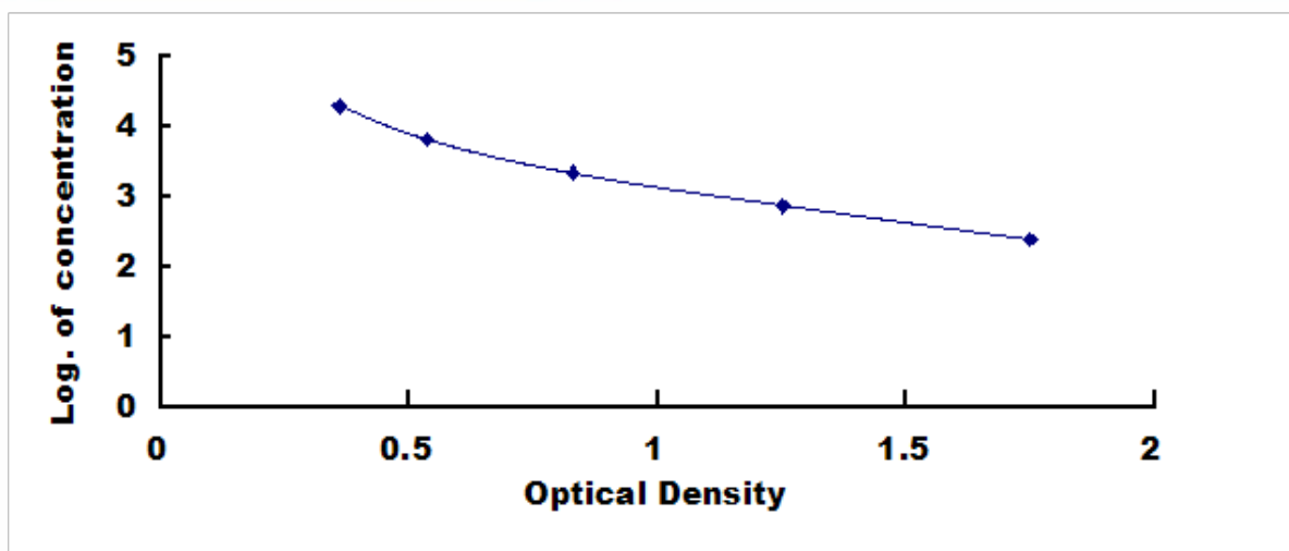
牛血清白蛋白 (BSA) 检测试剂盒标准曲线
