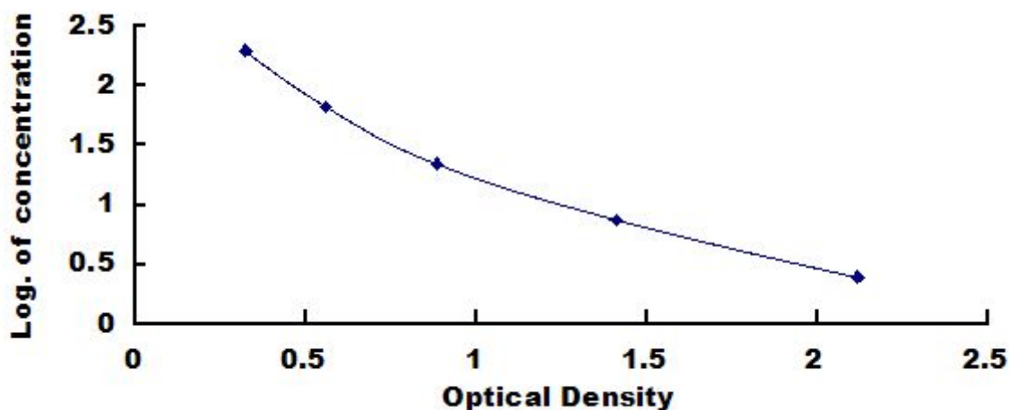
大鼠心肌肌钙蛋白 I (TNNT3) 检测试剂盒标准曲线
