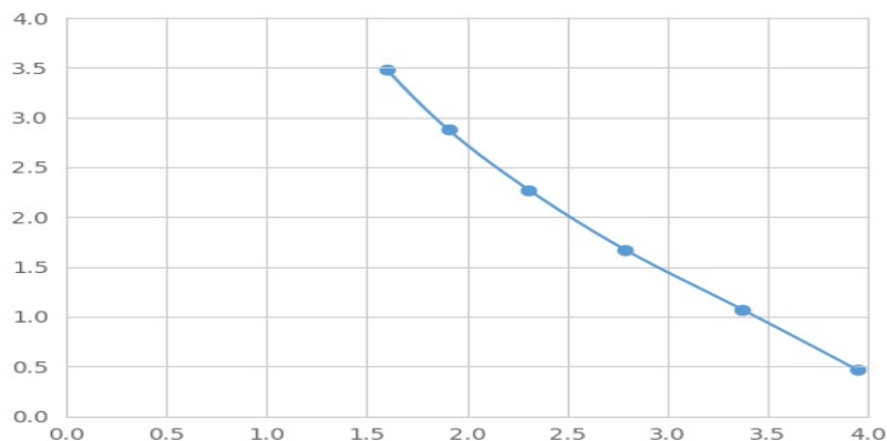
(β-黑素细胞刺激素)检测试剂盒标准曲线
