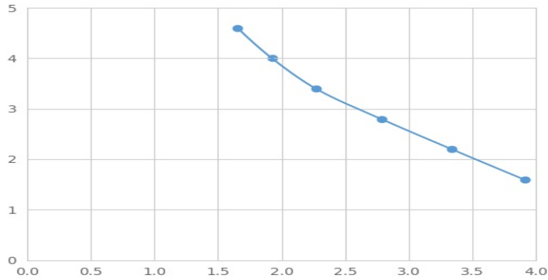
(钙泊三醇)检测试剂盒标准曲线
