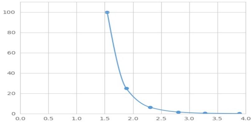
(瓜氨酸)检测试剂盒标准曲线
