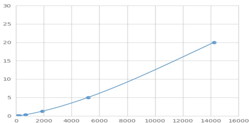
(糖蛋白 V) 检测试剂盒标准曲线
