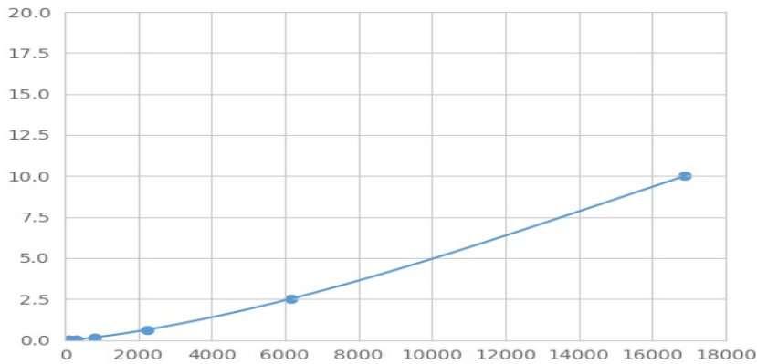
(外核苷三磷酸二磷酸水解酶1)检测试剂盒标准曲线
