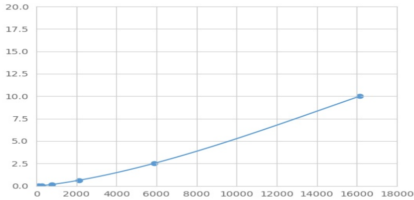
(葡萄糖6磷酸异构酶)检测试剂盒标准曲线
