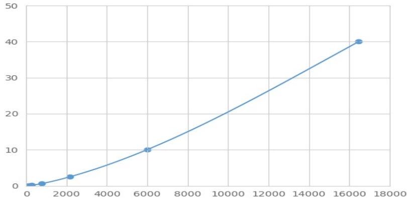
(细胞色素P450家族成员2C18)检测试剂盒标准曲线
