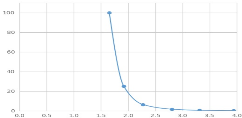
(左炔诺孕酮)检测试剂盒标准曲线
