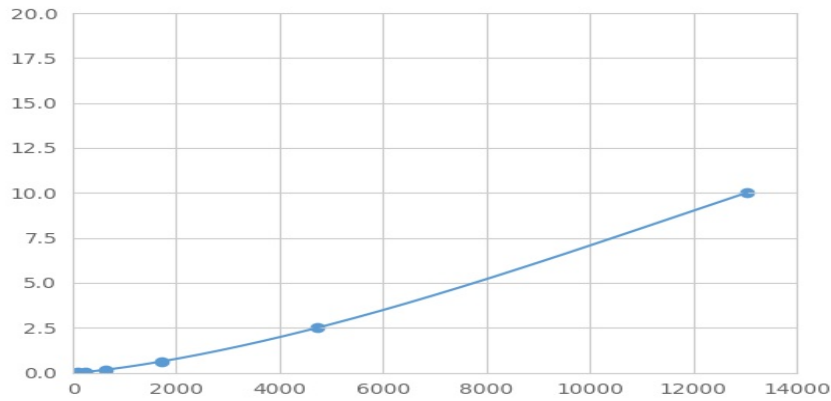
(N-甲基嘌呤DNA糖基化酶)检测试剂盒标准曲线
