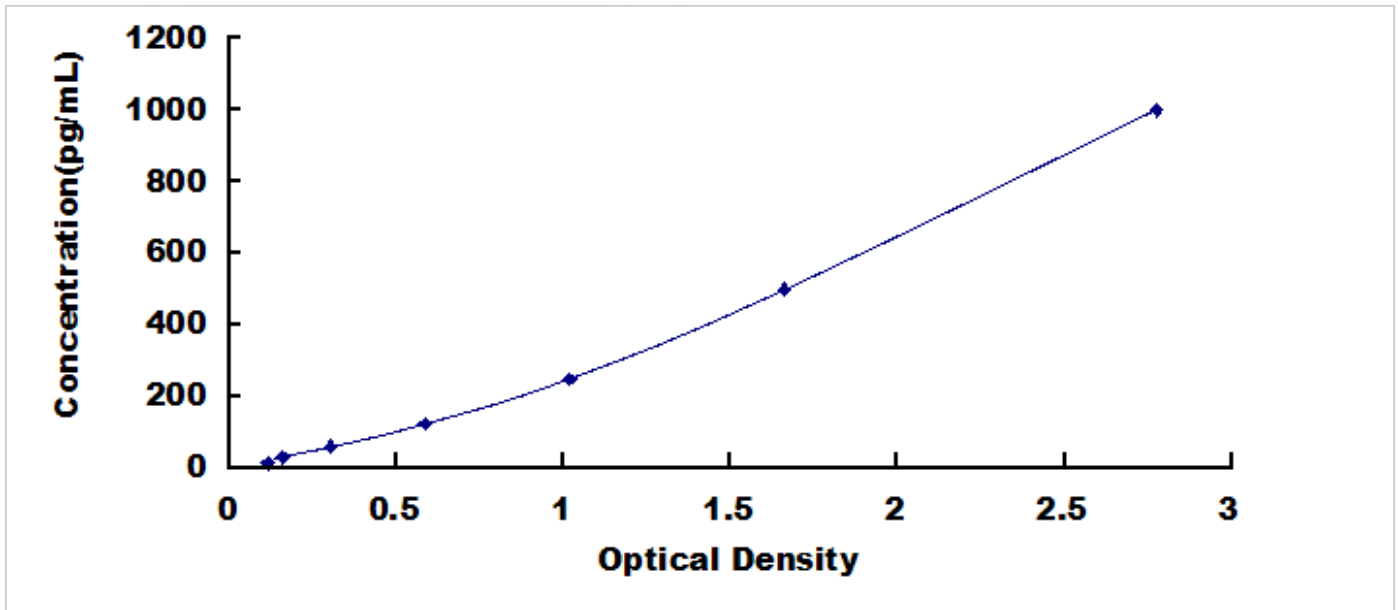
人白介素 12(IL12) 检测试剂盒标准曲线
