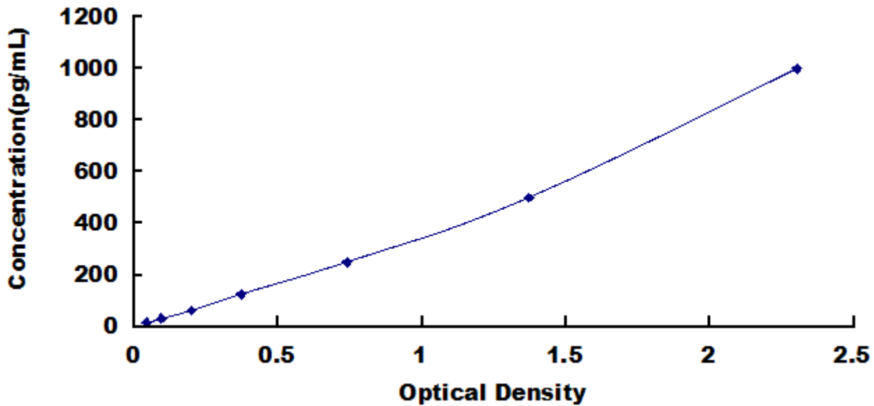
人白介素 27 (IL27) 检测试剂盒标准曲线
